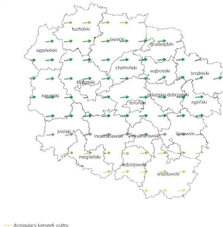
Rysunek 6. Dominujący kierunek wiatru wyznaczony przez model WRF/CALMET w strefie kujawsko-pomorskiej w 2015 r.
